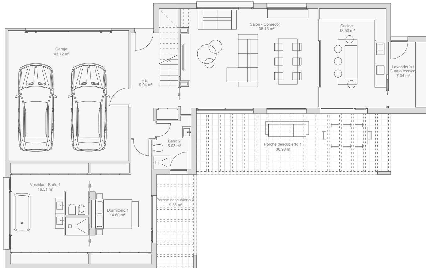
PLANTA BAJA
