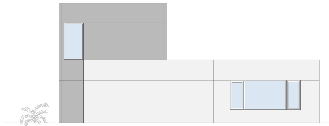
ALZADO B
