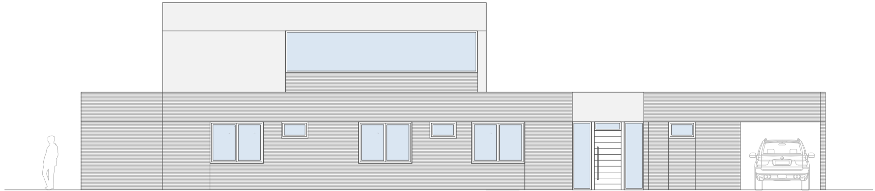
ALZADO A
