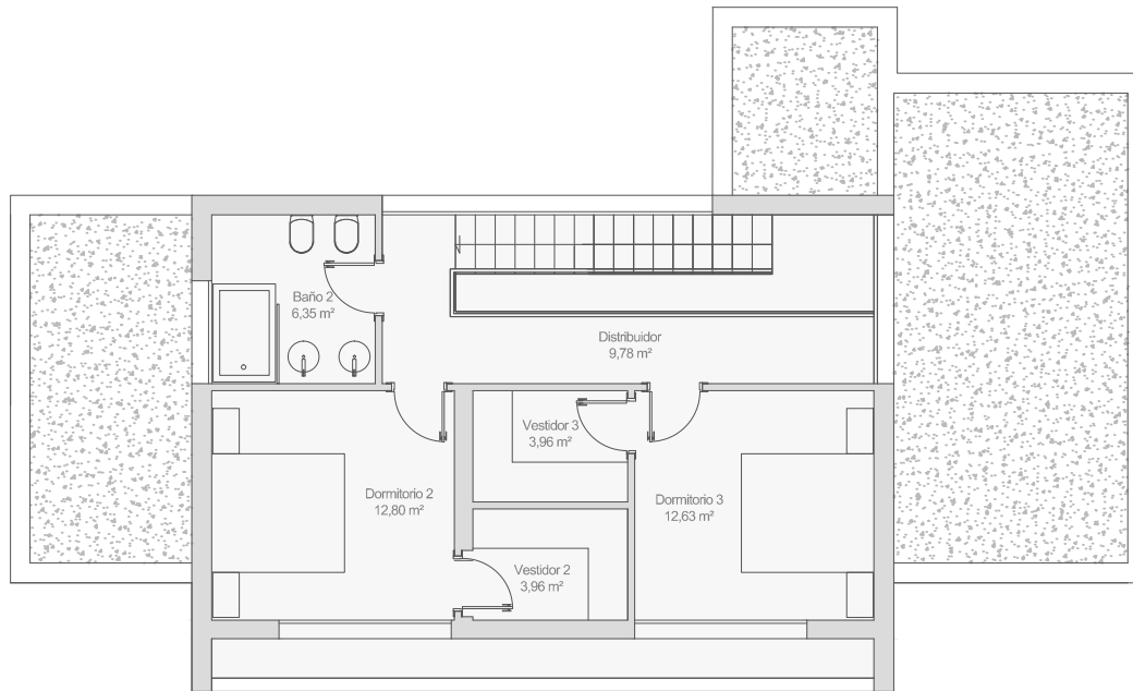
PLANTA ALTA
